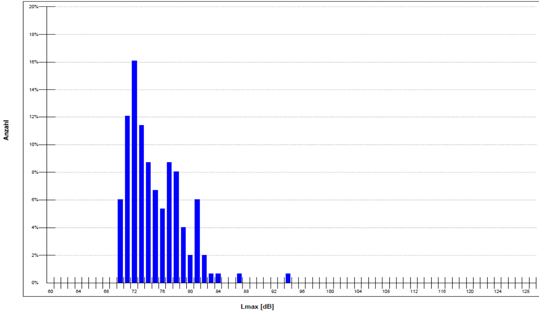
Maximalpegel-Verteilung korr. Lärmereignisse MP04 im Mai 2014
